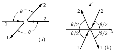
图 16.2: 两个以相等速率、相向运动的相同粒子所发生的弹性碰撞的两种视图
