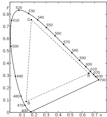
图 35.4: 标准色品图
